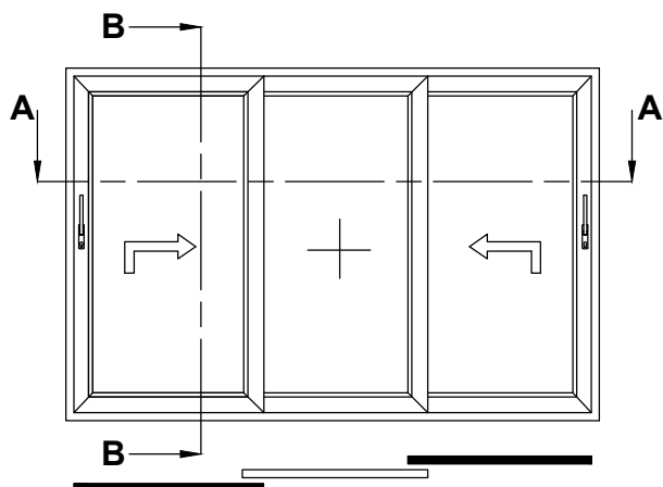
Schema C
