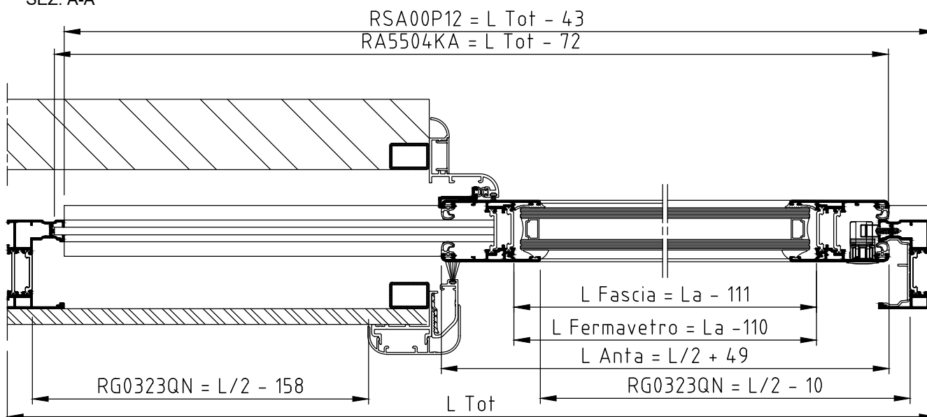
SEZ. A-A
