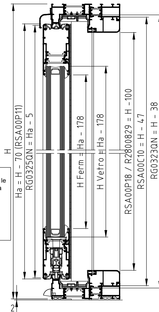
SEZ. B-B
