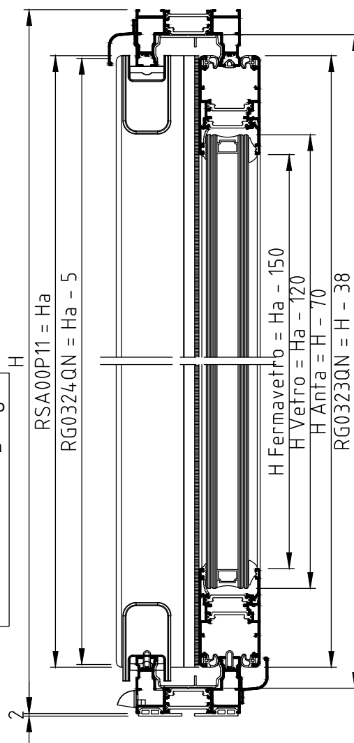
SEZ. B-B
