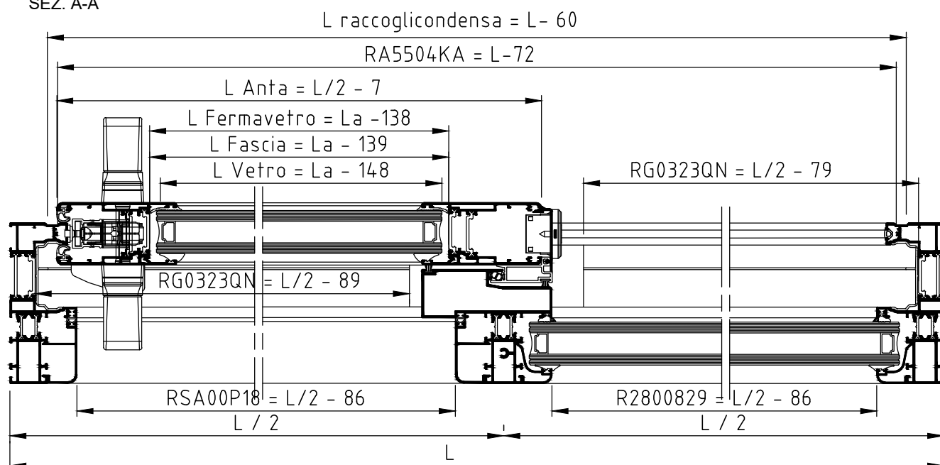
SEZ. A-A
