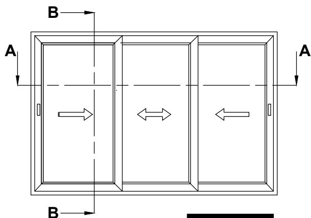
Schema D
