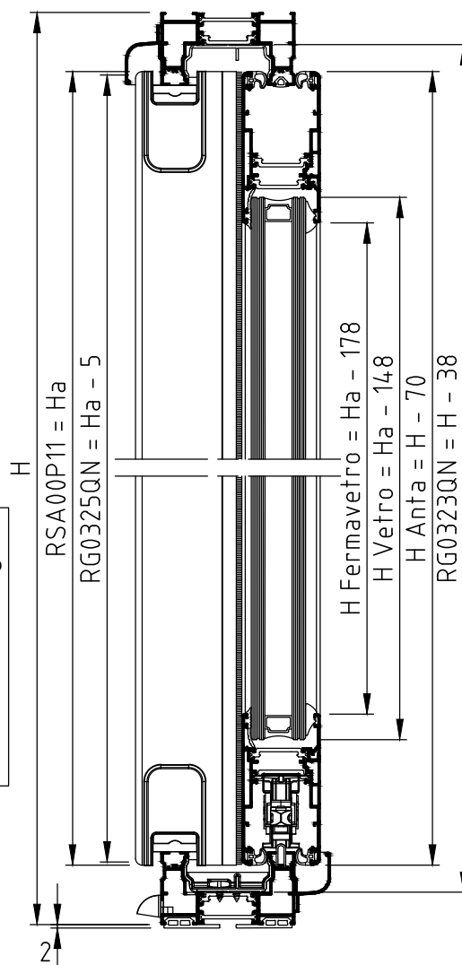
SEZ. B-B
