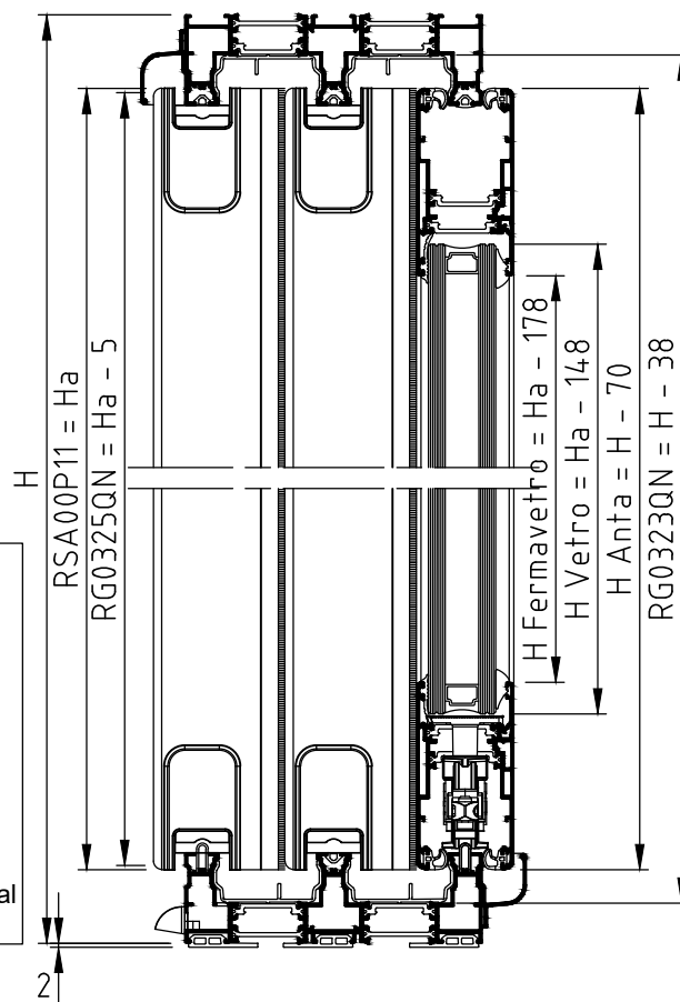
SEZ. B-B
