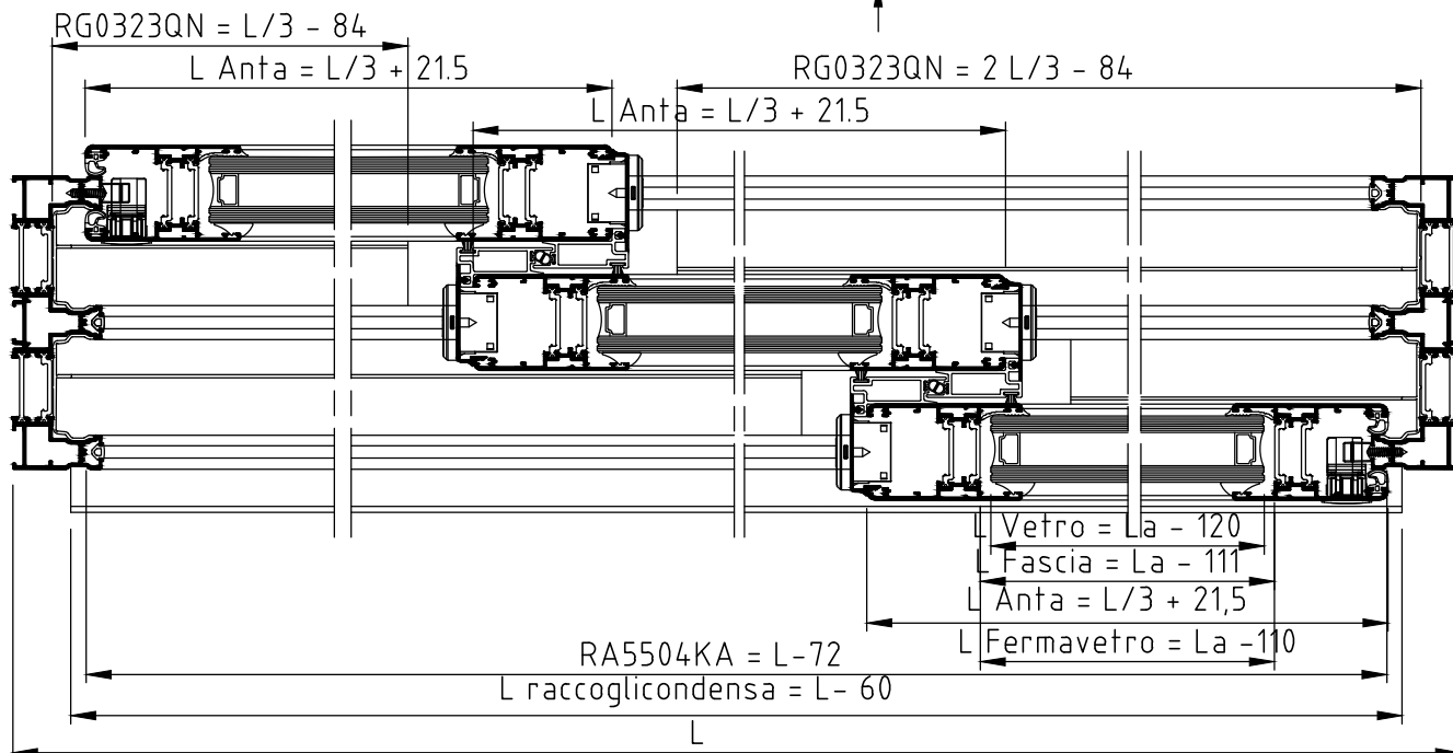
SEZ. A-A
