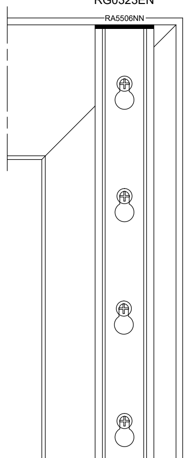
Vista C-C
