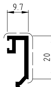
FERMAVETRO GLAZING BEAD
