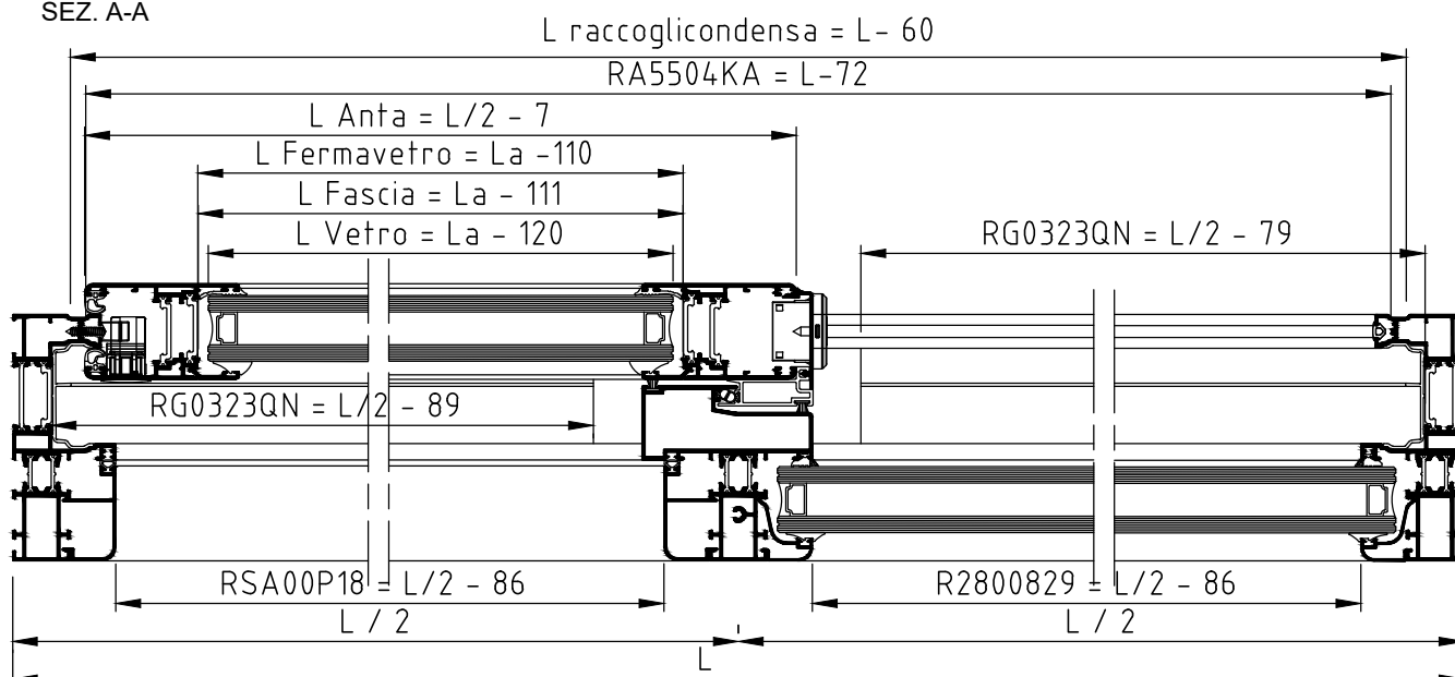
SEZ. A-A
