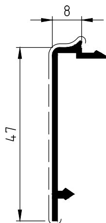
CARTELLINA PER ANTE SASH CARTER
